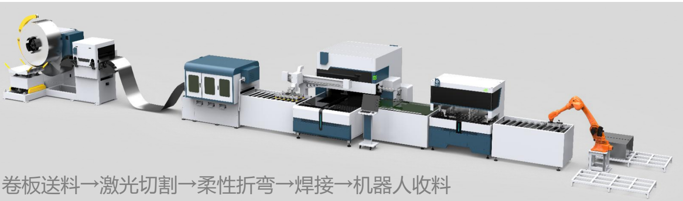
华北区首条钢制家具自动化生产线
